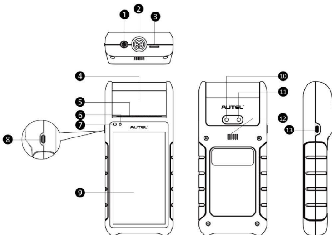
Рисунок 2-1. Внешний вид диагностического сканера MaxiBAS VT608 (виды спереди, сзади и сбоку)
